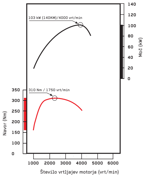
2.0 litrski DI-D s filtrom trdnih delcev (DPF)
