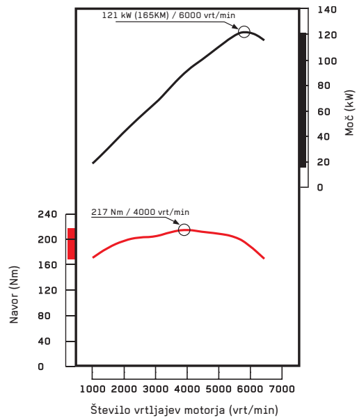
2.4 litrski MIVEC
